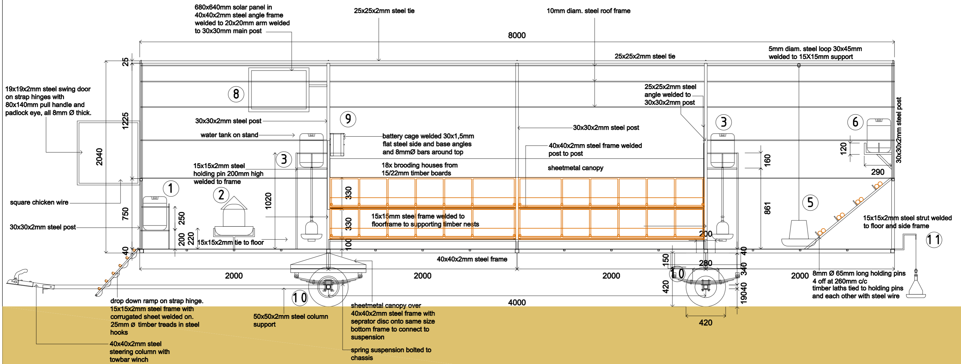
EGG MOBILE Longitudinal Section 1 : 25
